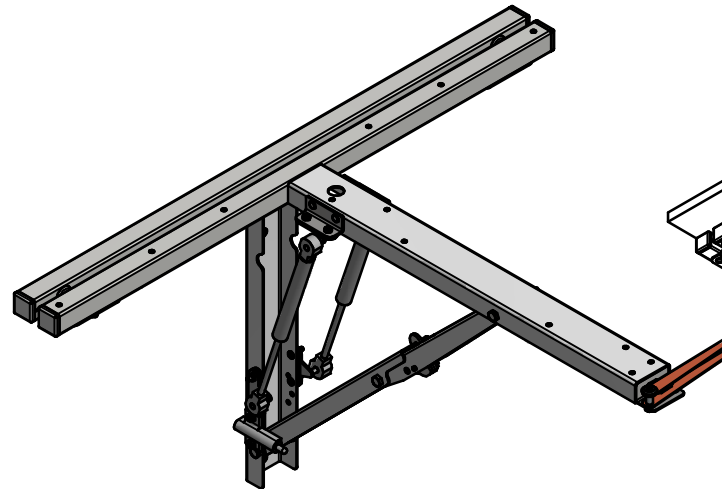
Установка столешницы
