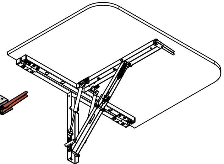
Установка столешницы
